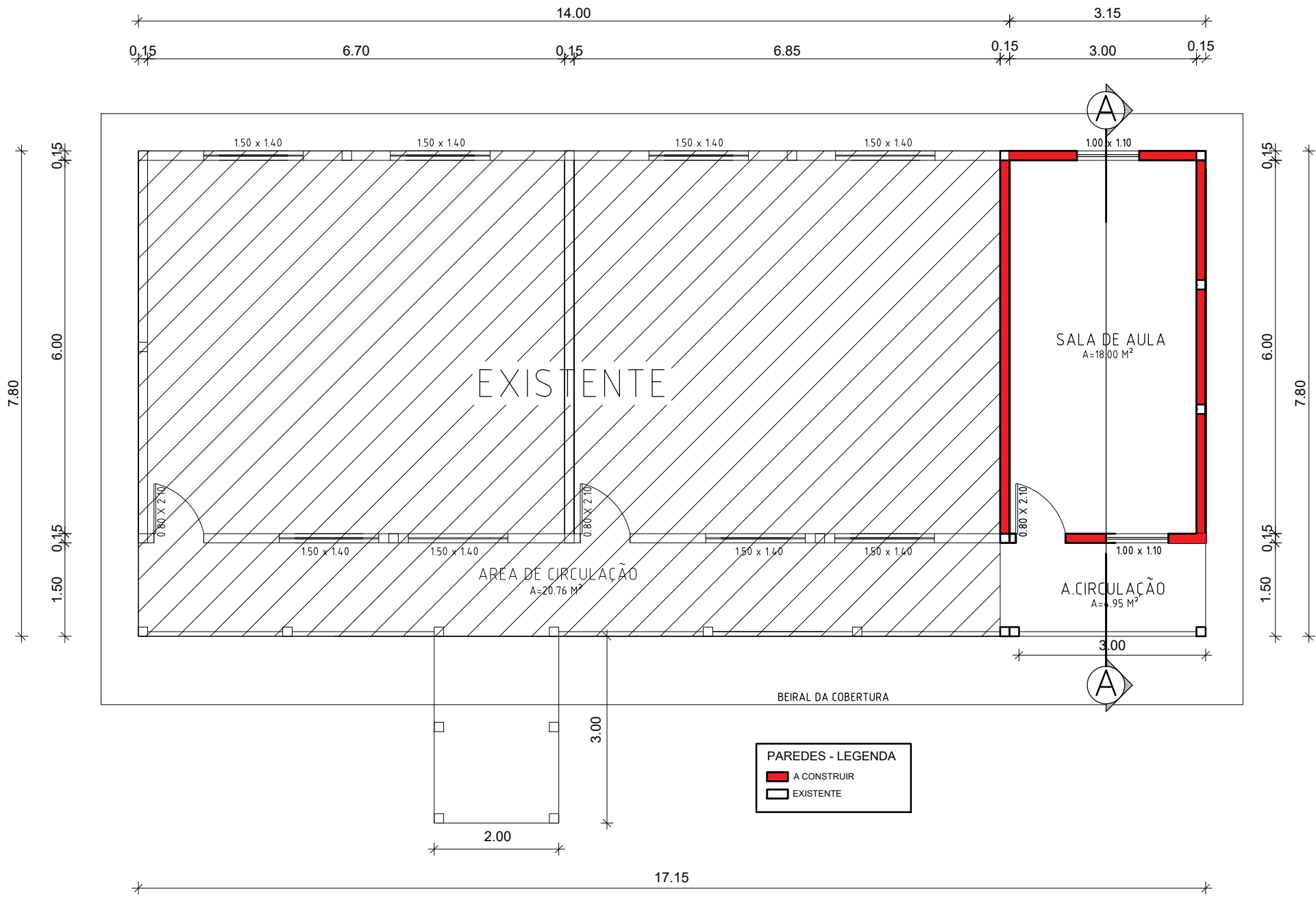
PLANTA BAIXA - FRANCISCO NAPOLEÃO DE ARAÚJO S/ESCALA
