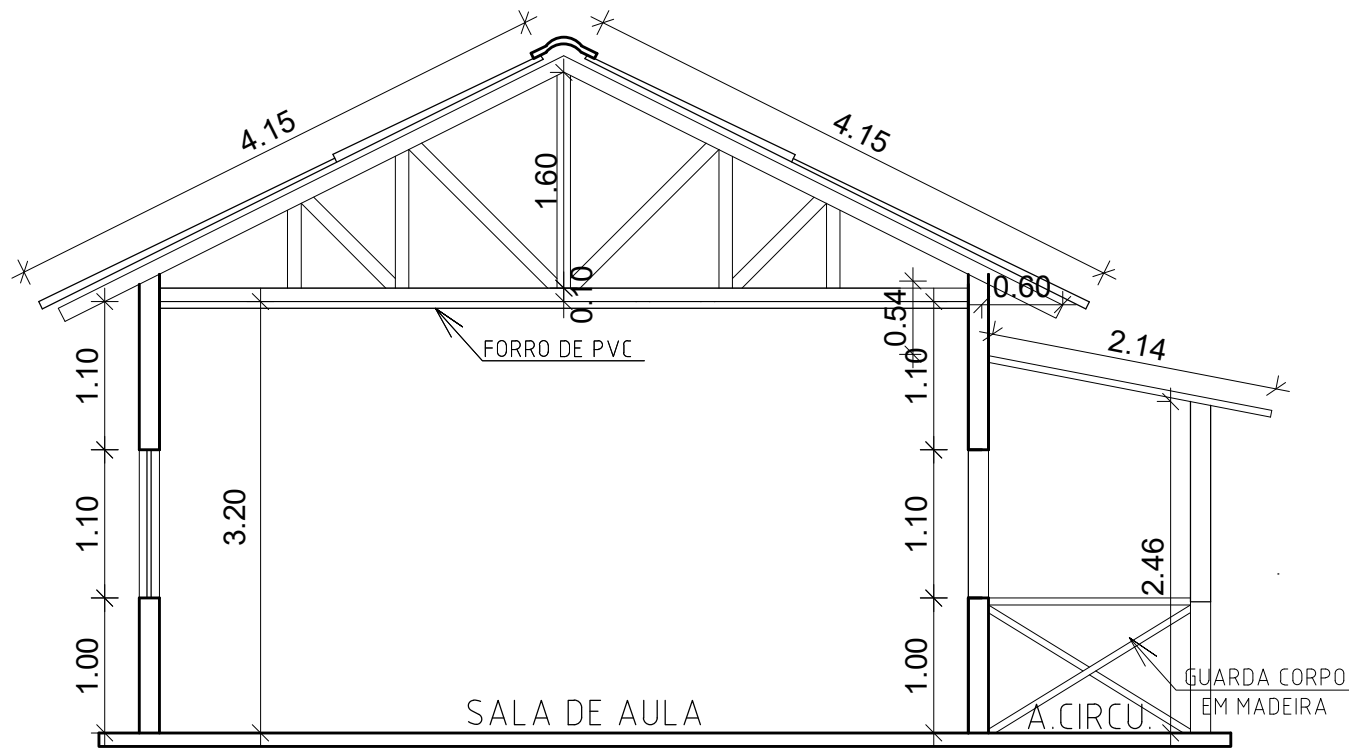
CORTE AA - FRANCISCO NAPOLEÃO ARAÚJO SEM ESCALA
